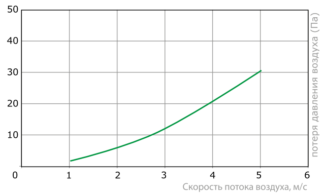
Аэродинамическое сопротивление клапанов воздушных V.1 и обратных VO.1
