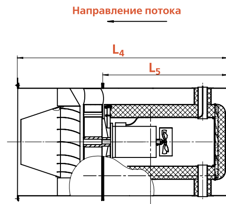
SHAULA SE.400 AX.S.SA SHAULA SE.600 AX.S.SA
