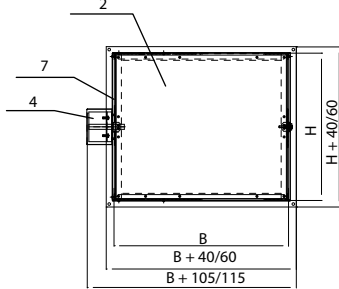
Клапан канальный 120 мин НО/НЗ
