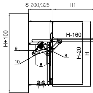
Клапан дымовой 90/120/180 мин
