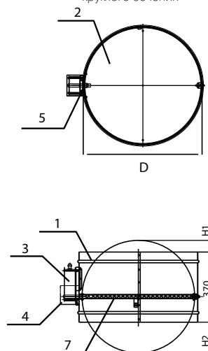
Клапан канальный 90 мин НО/НЗ круглого сечения
