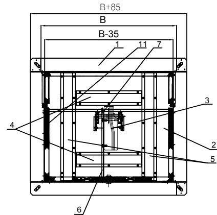
Клапан дымовой 90/120/180 мин
