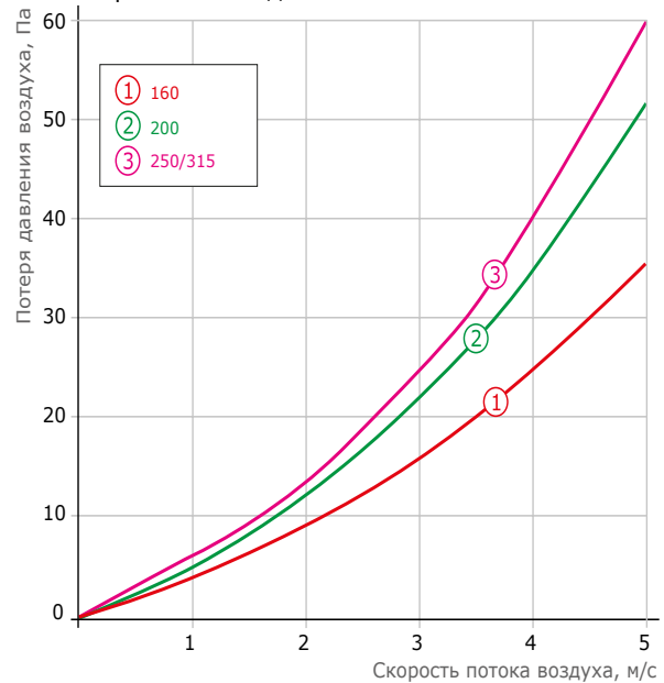
Аэродинамическое сопротивление нагревателей водяных HW.
