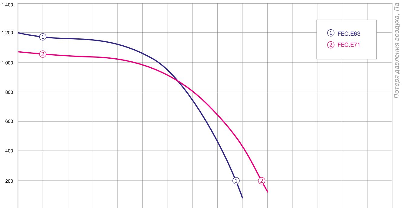
Расход воздуха (в зависимости от числа модулей в решении MULTI-FAN), м³/ч
