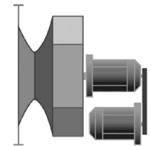
/FRRH. Вентилятор «свободное колесо», «горячий» резерв
