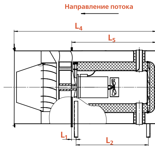
SHAULA SE.400 AX.F.SA SHAULA SE.600 AX.F.SA
