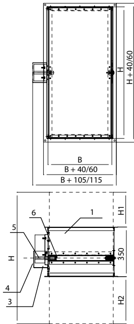
Клапан каналный 60 мин НО/НЗ прямоугольного сечения
