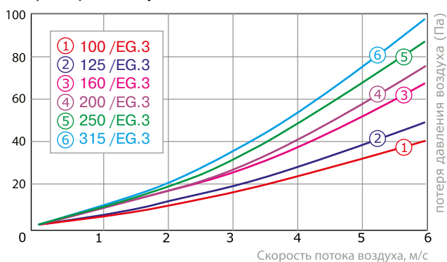
Аэродинамическое сопротивление фильтров воздушных EG.3
