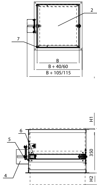
Клапан каналный 60 мин с ТЗ
