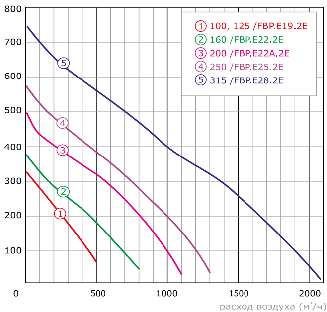
Аэродинамические характеристики вентиляторов /FB_.
