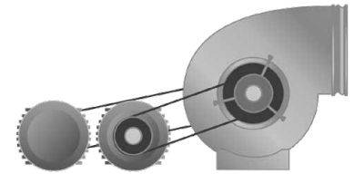
/FDRH. Вентилятор двустороннего всасывания, «горячий» резерв
