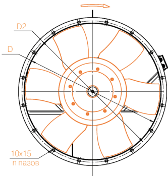
Исполнение AX.F Направление вращения
