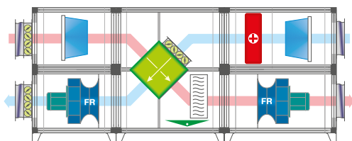
SIRIUS ST 280 LR //G.(EG.-HW.)[RX.=RX.][FR.]V.-G./G.-V.(EG.)[FR.]G.
