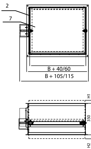
Клапан канальный 90 мин НО/НЗ прямоугольного сечения
