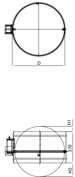
Клапан каналный 60 мин НО/НЗ круглого сечения
