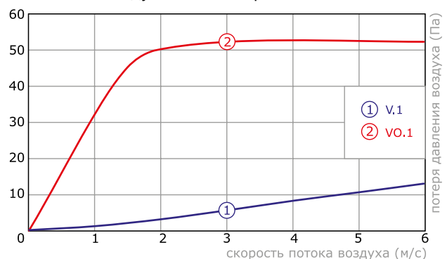
Аэродинамическое сопротивление клапанов воздушных V.1 и обратных VO.1
