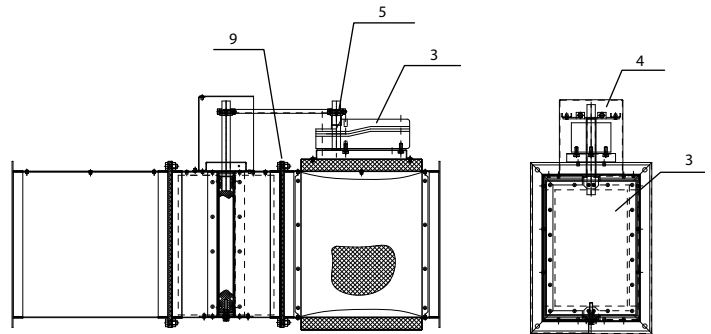
Клапан канальный 120 мин двойного действия
